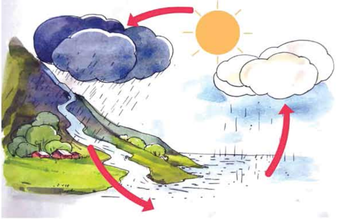
চিত্র: পানিচক্র
